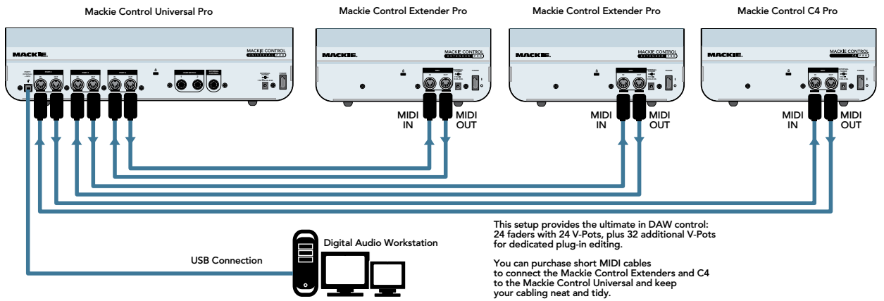
Hookup 1: USB
