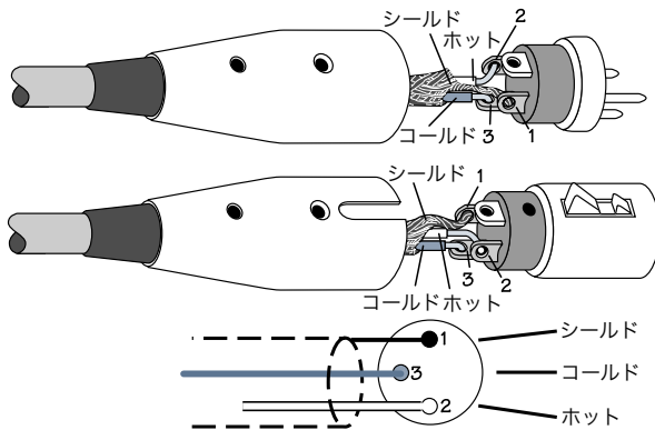
バランスXLRコネクタ
