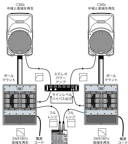
2 × SWA1801z + ステレオアンプ + 2 × C300z
