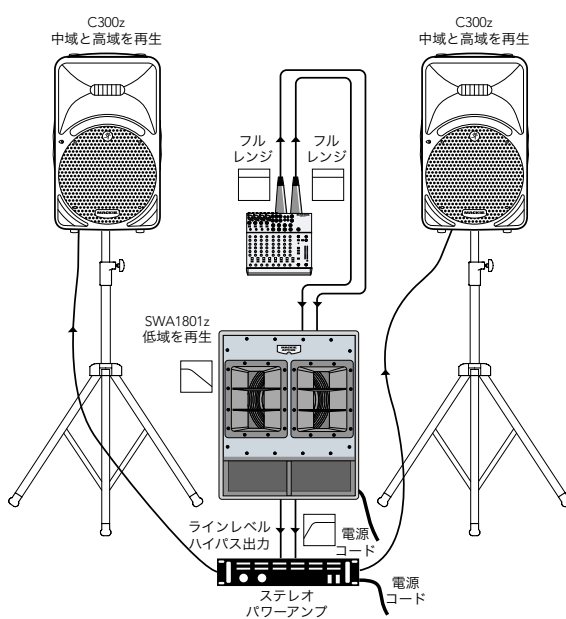
SWA1801z + ステレオアンプ + 2 × C300z
